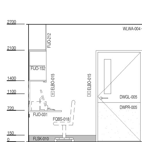
ELEVATION 3
