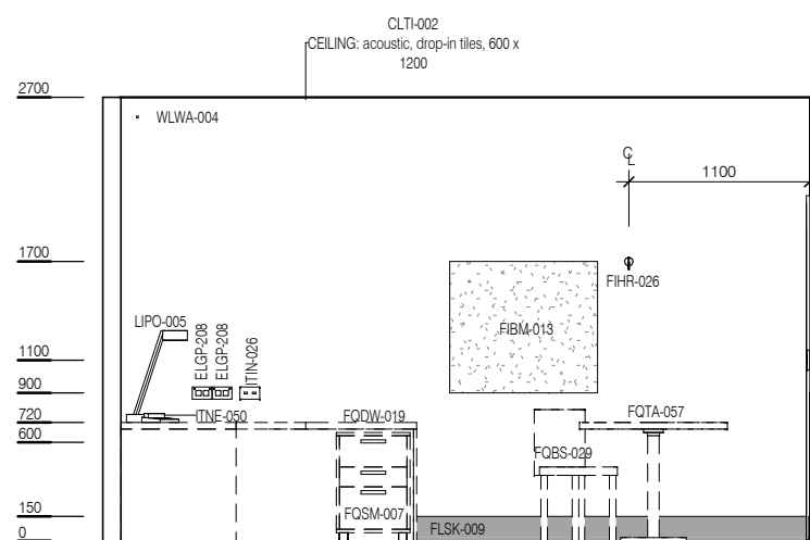
ELEVATION 2
