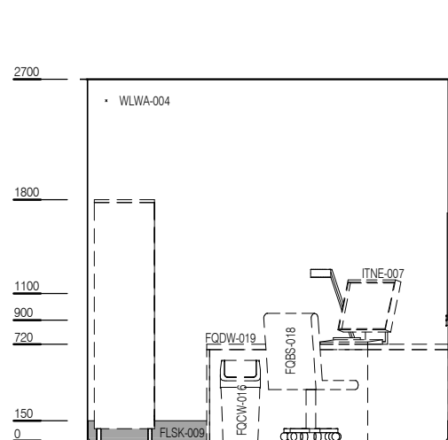
ELEVATION 1
