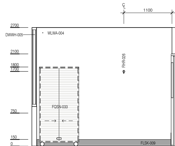
ELEVATION 2
