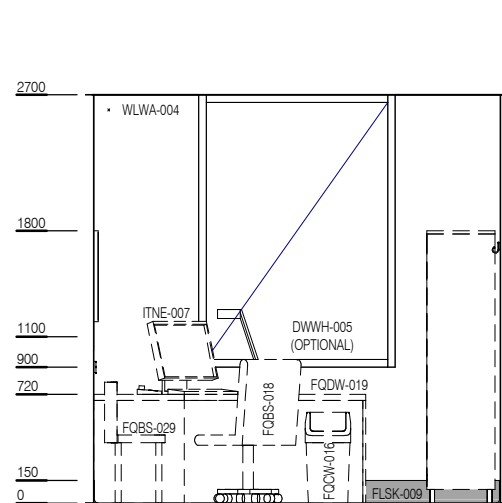
ELEVATION 1
