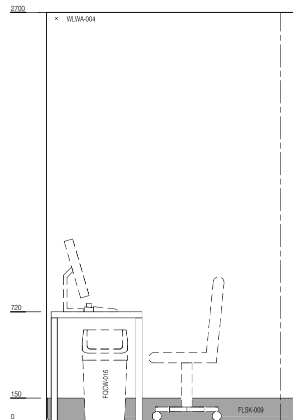
ELEVATION 1
