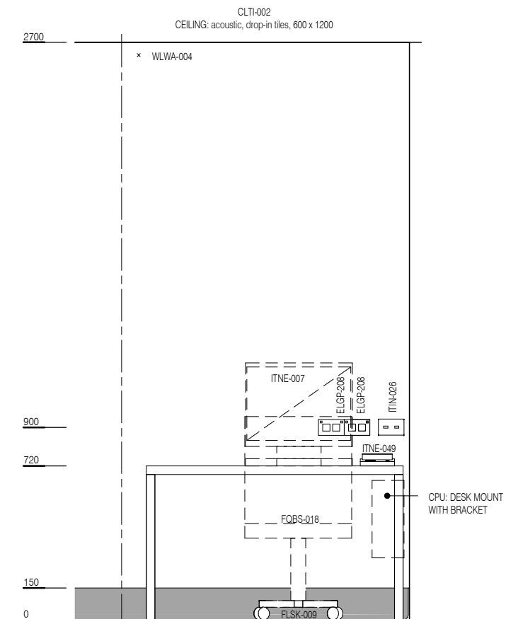
ELEVATION 2
