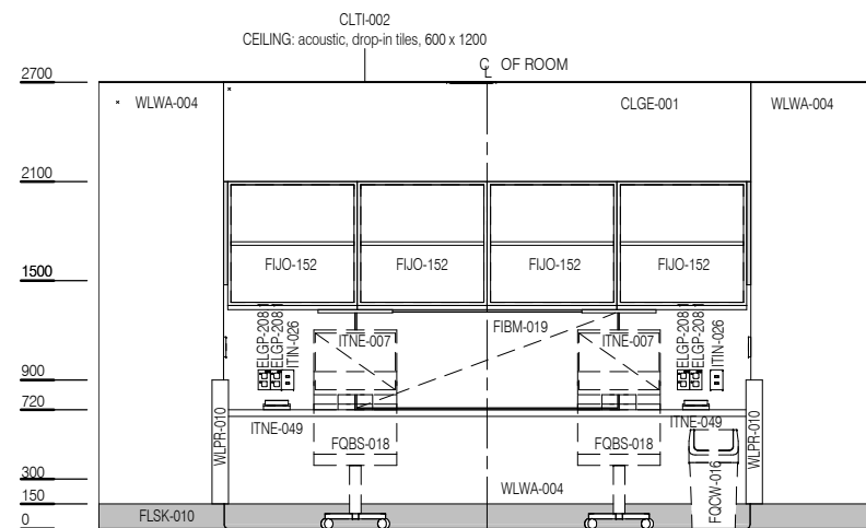
ELEVATION 2
