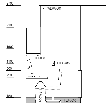
ELEVATION 3
