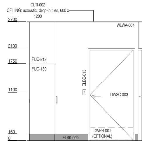
ELEVATION 3
