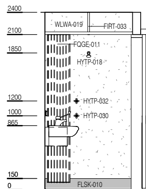
ELEVATION 1
