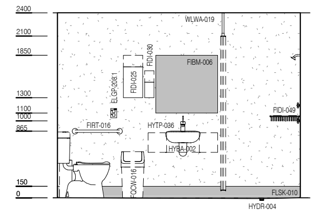
ELEVATION 4
