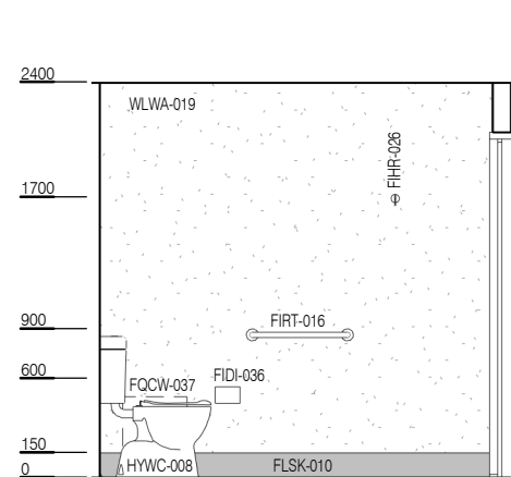
ELEVATION 1
