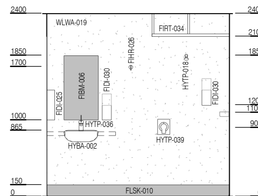
ELEVATION 3
