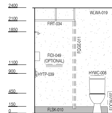
ELEVATION 4
