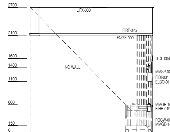
ELEVATION 3
