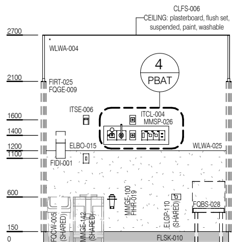
ELEVATION 1
