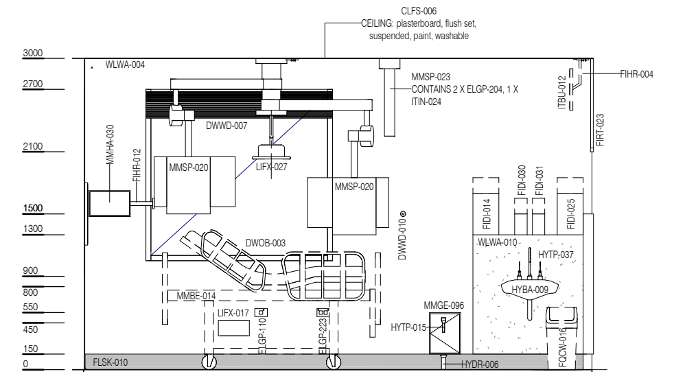
ELEVATION 2
