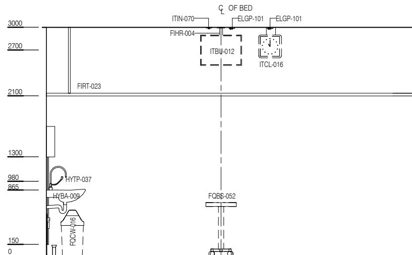
ELEVATION 3
