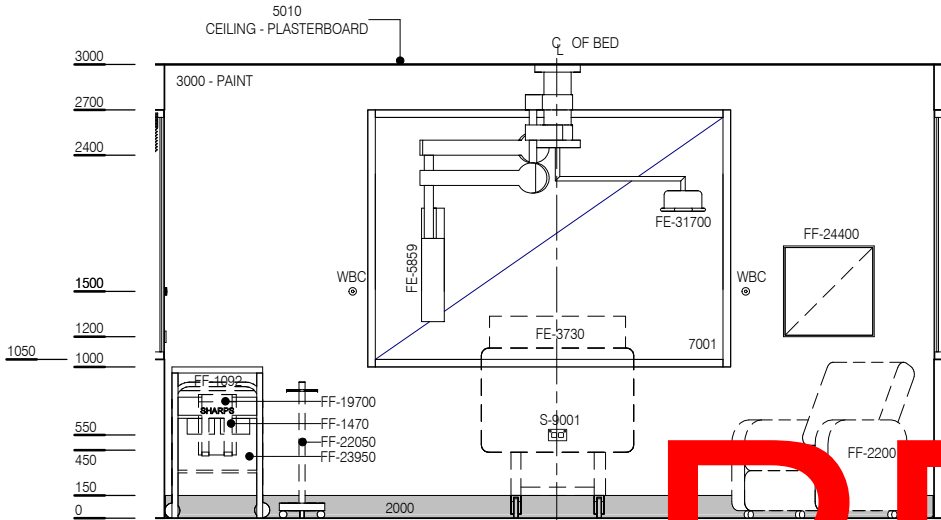
ELEVATION 1
