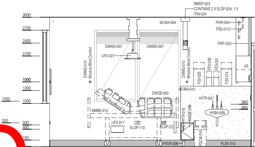
ELEVATION 2
