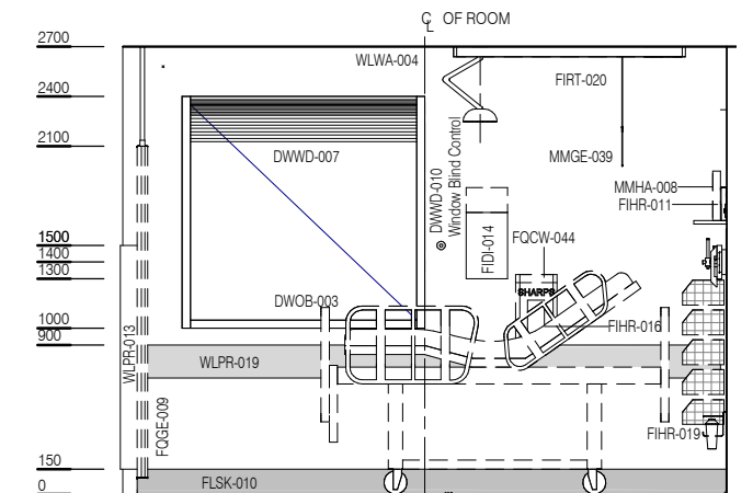
ELEVATION 4
