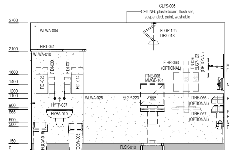
ELEVATION 4
