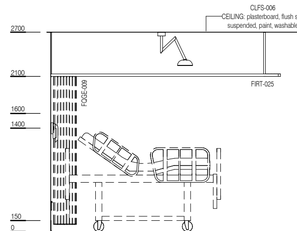
ELEVATION 2
