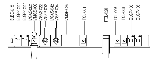
ELEVATION 3
