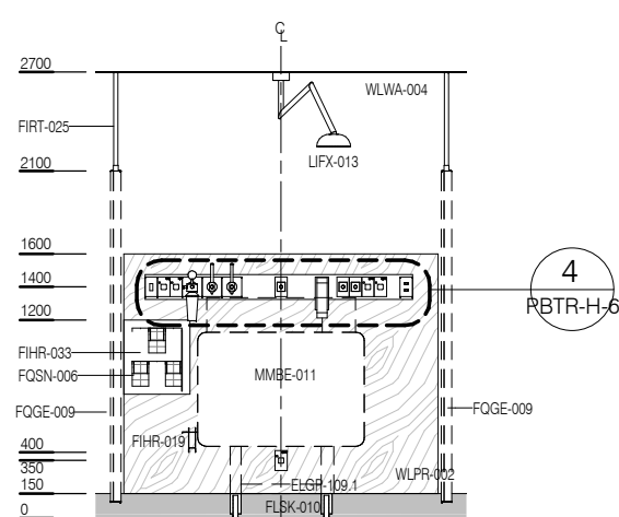
ELEVATION 1
