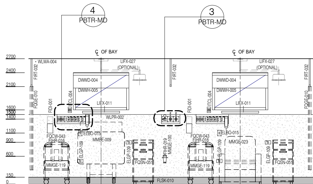
ELEVATION 1
