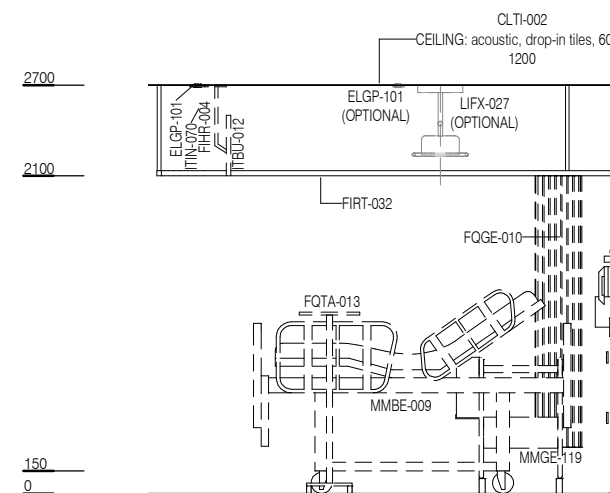
ELEVATION 2
