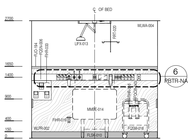
ELEVATION 1
