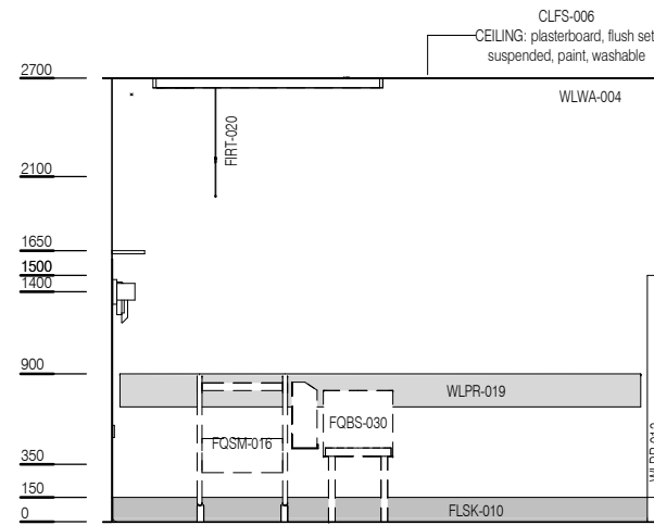
ELEVATION 2
