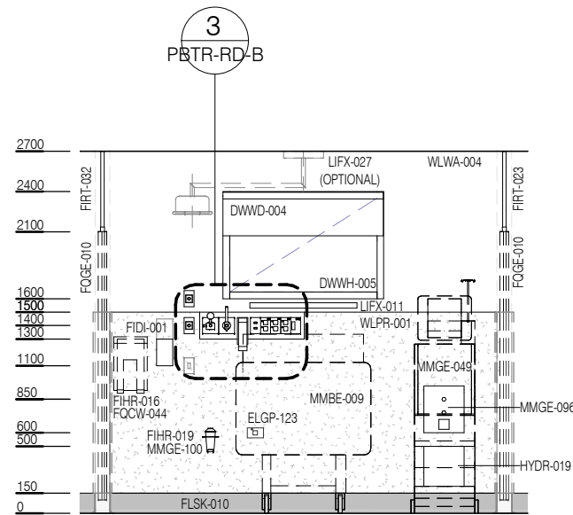
ELEVATION 1
