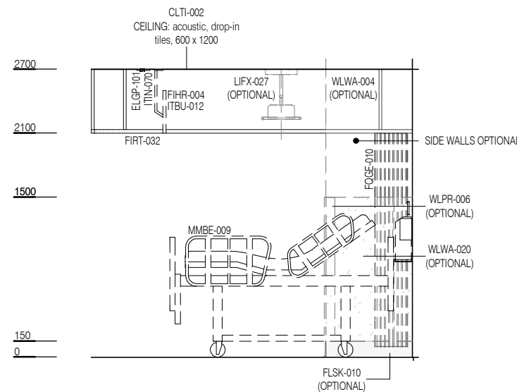
ELEVATION 2
