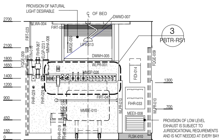
ELEVATION 1
