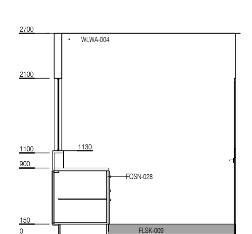
ELEVATION 4
