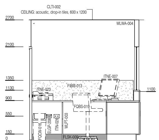
ELEVATION 2
