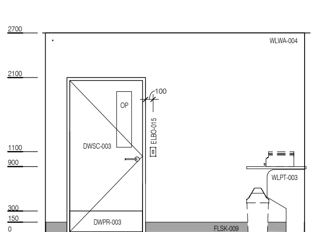
ELEVATION 1
