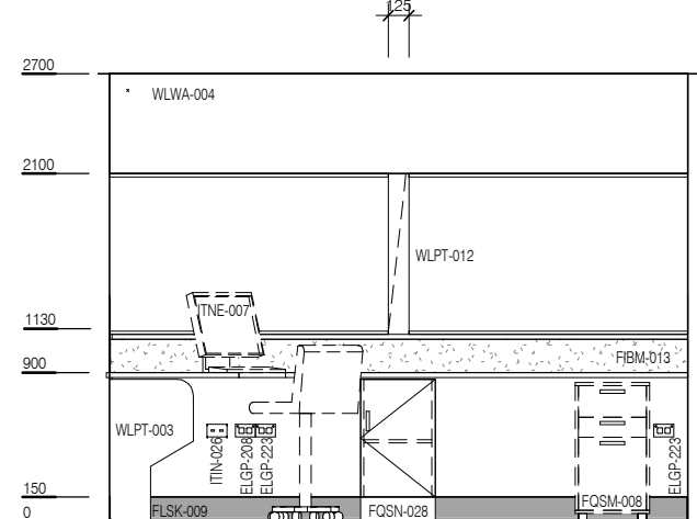
ELEVATION 3
