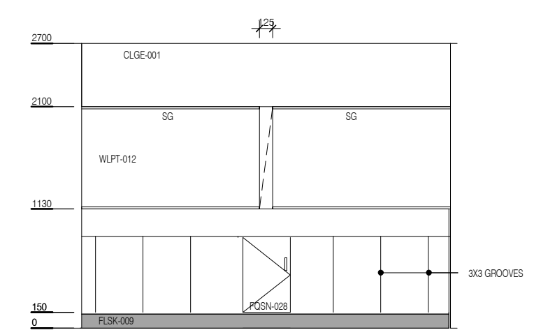
ELEVATION 5
