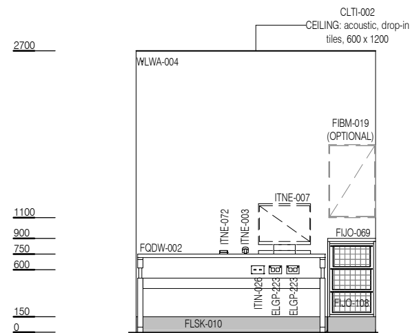
ELEVATION 2
