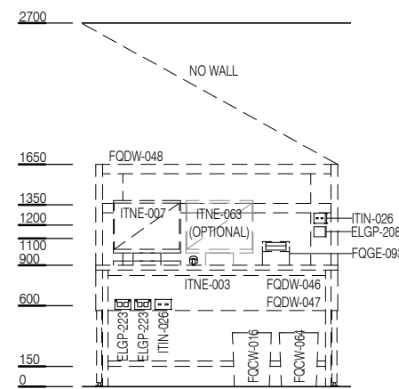
ELEVATION 2
