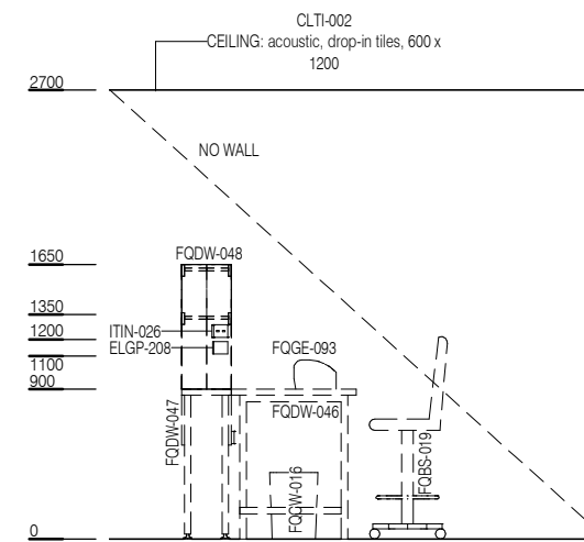
ELEVATION 3
