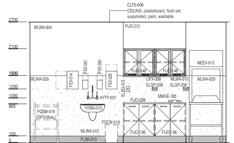
ELEVATION 4
