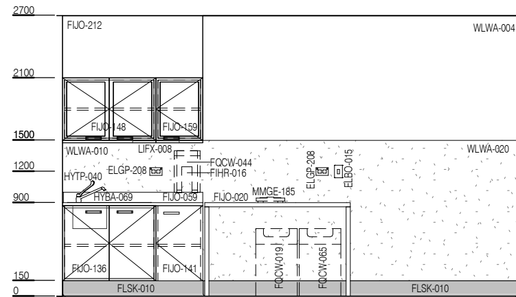
ELEVATION 2
