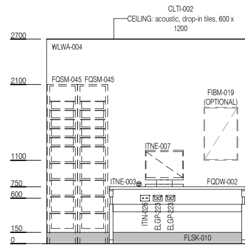
ELEVATION 2
