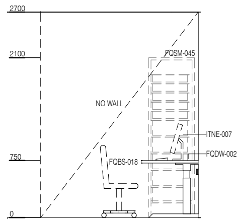
ELEVATION 1
