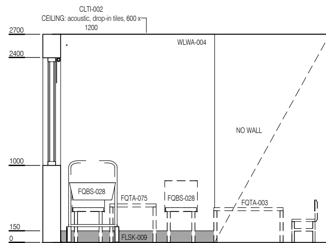
ELEVATION 2
