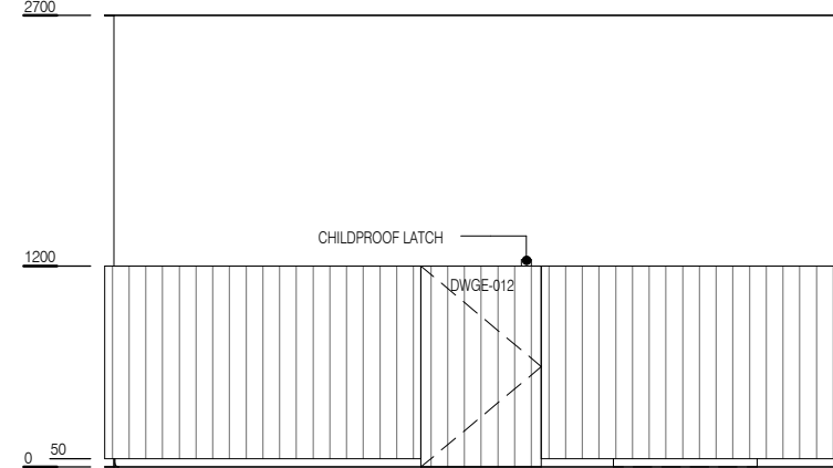
ELEVATION 3
