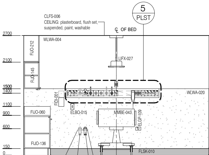
ELEVATION 1
