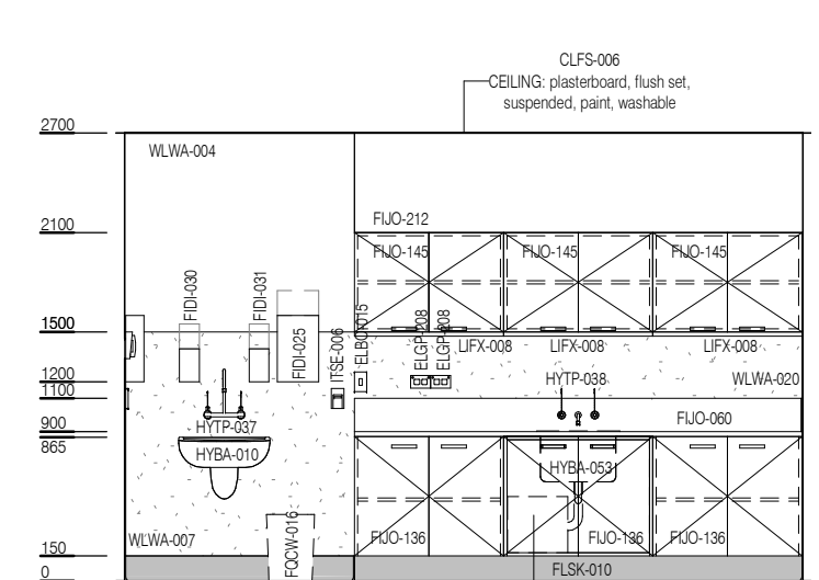
ELEVATION 4
