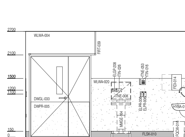
ELEVATION 3
