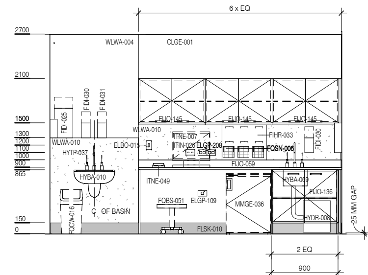
ELEVATION 4
