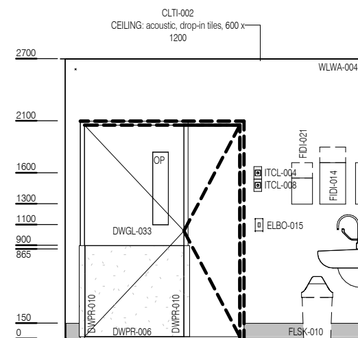
ELEVATION 3
