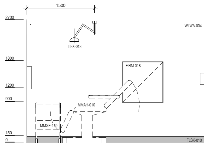
ELEVATION 2
