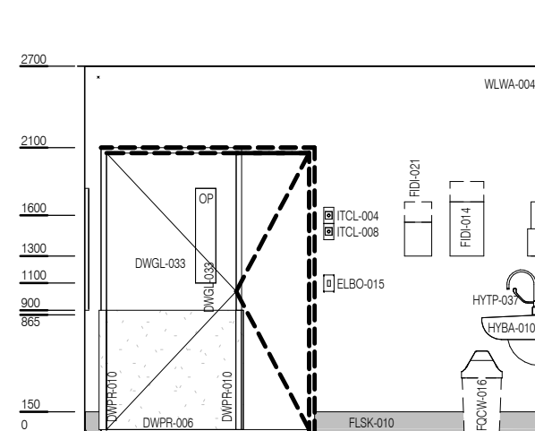
ELEVATION 3
