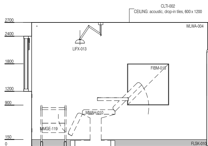
ELEVATION 2
