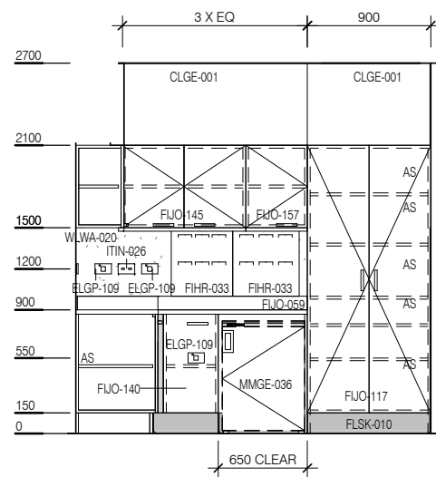
ELEVATION 1
