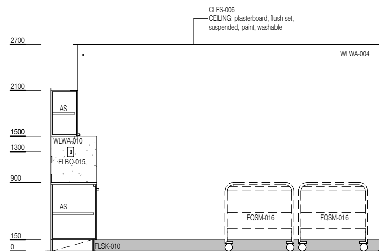
ELEVATION 2
