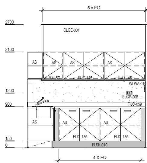
ELEVATION 1
