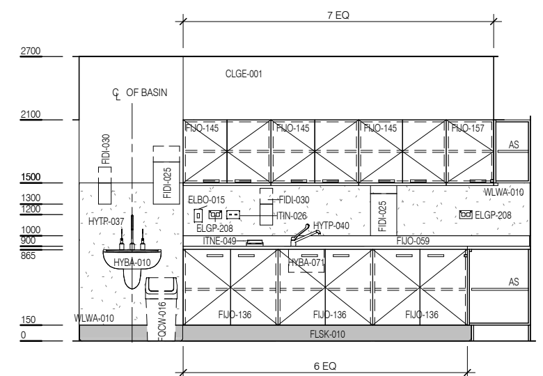
ELEVATION 4
