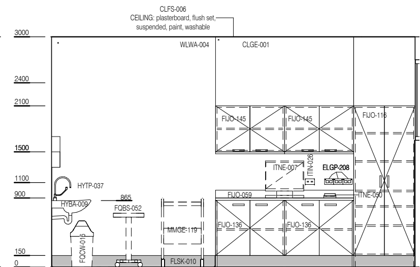
ELEVATION 4
