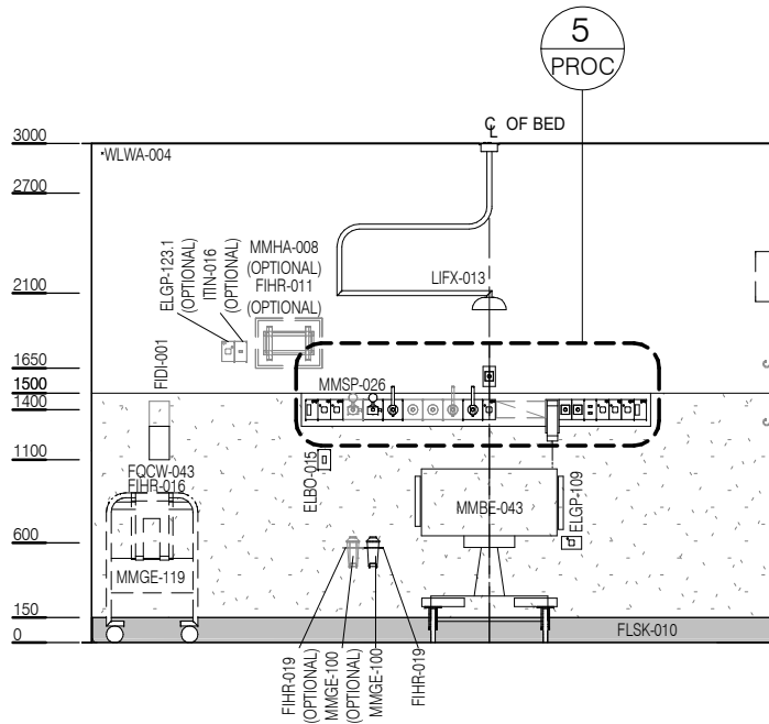
ELEVATION 1
