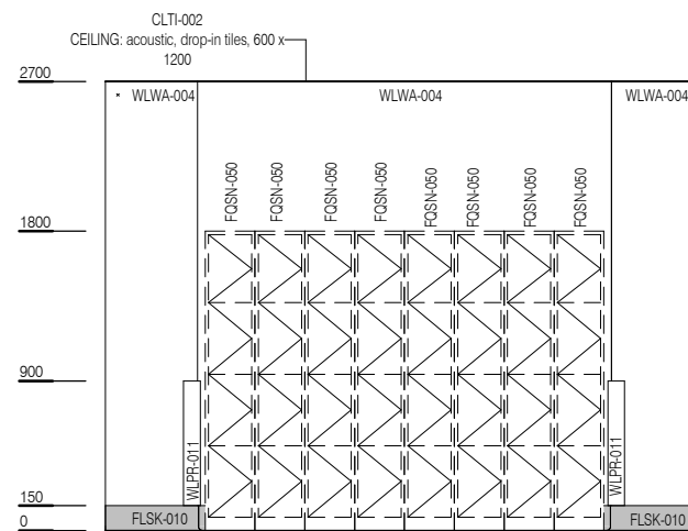
ELEVATION 2
