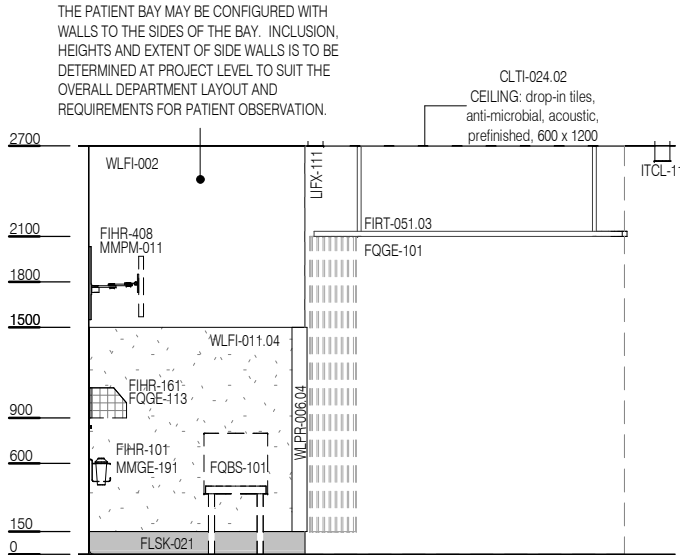
ELEVATION 3
