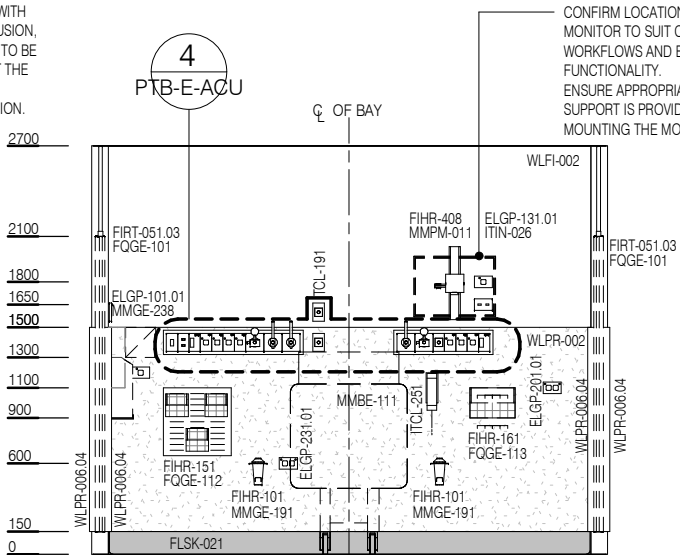
ELEVATION 2
