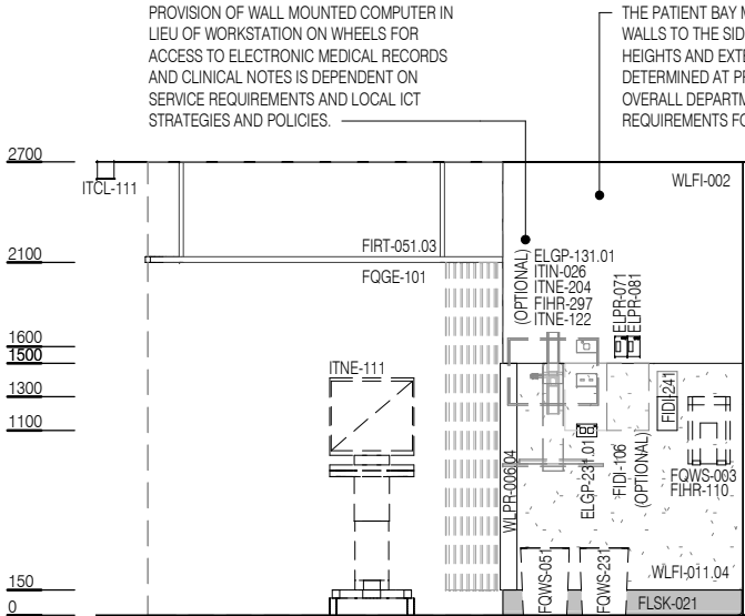
ELEVATION 1
