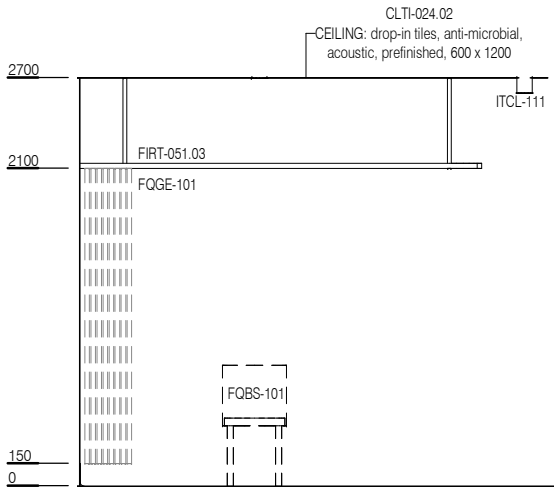
ELEVATION 3
