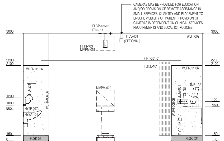
ELEVATION 4
