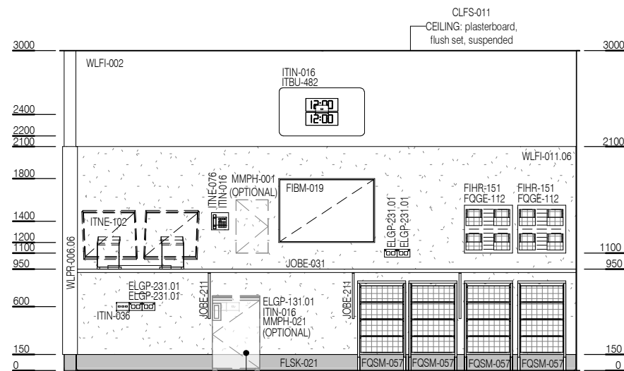
ELEVATION 1
