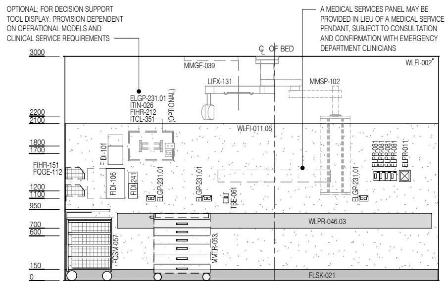
ELEVATION 2
