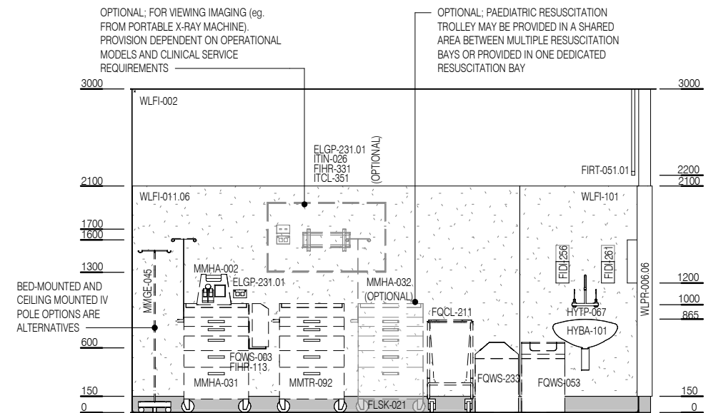
ELEVATION 3
