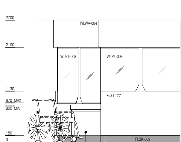
ELEVATION 1
