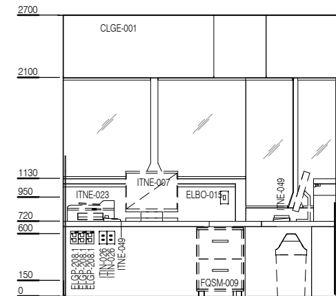
ELEVATION 3
