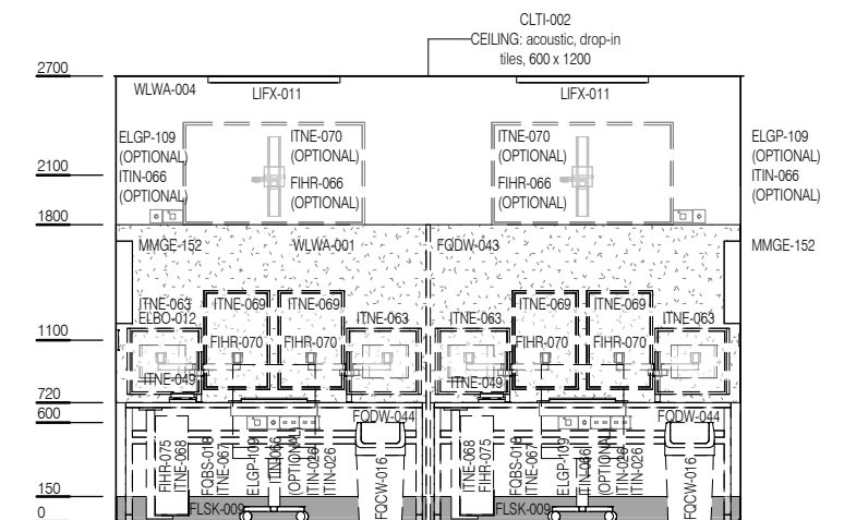
ELEVATION 4
