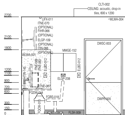
ELEVATION 1
