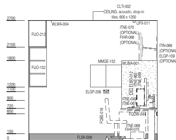
ELEVATION 3
