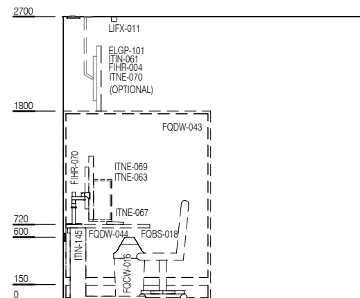
ELEVATION 2
