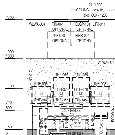
ELEVATION 1
