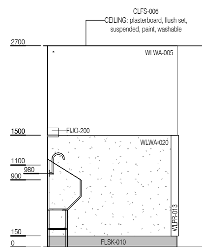
ELEVATION 2
