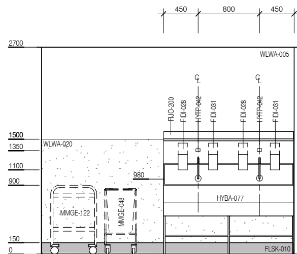
ELEVATION 1
