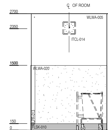
ELEVATION 3
