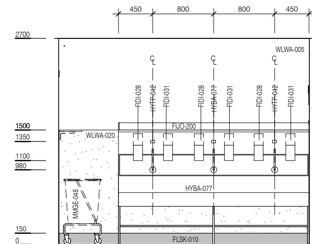
ELEVATION 4
