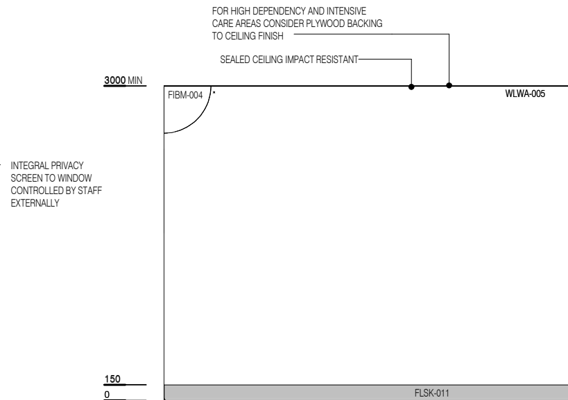
ELEVATION 5
