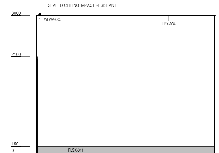
ELEVATION 4
