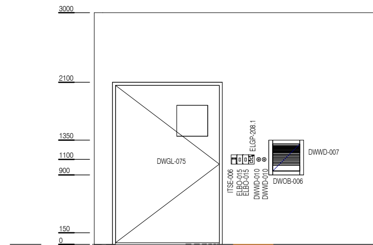
ELEVATION 5
