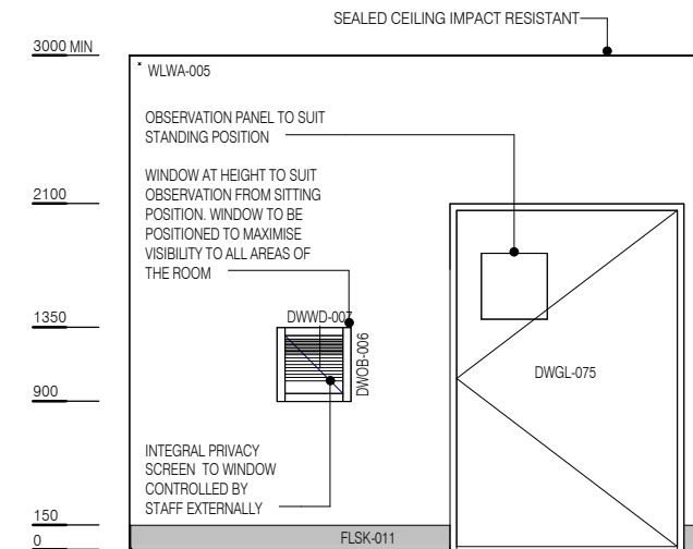
ELEVATION 3
