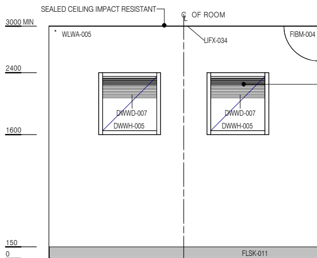
ELEVATION 1
