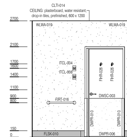
ELEVATION 4
