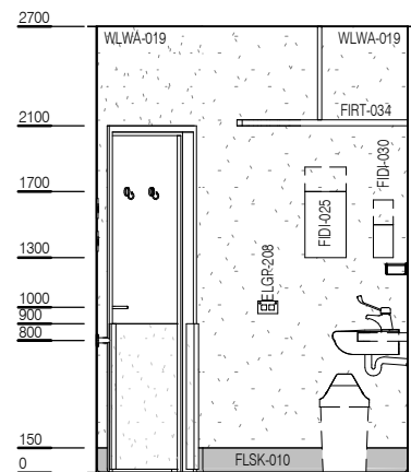
ELEVATION 1
