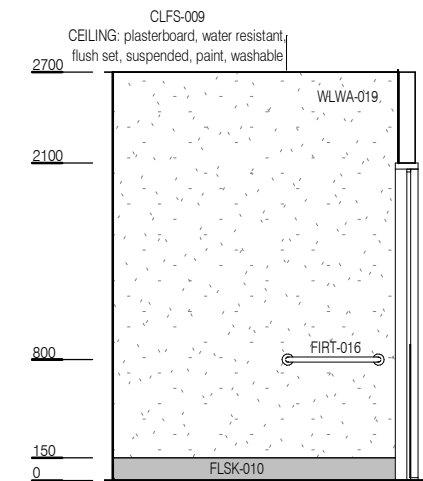
ELEVATION 4
