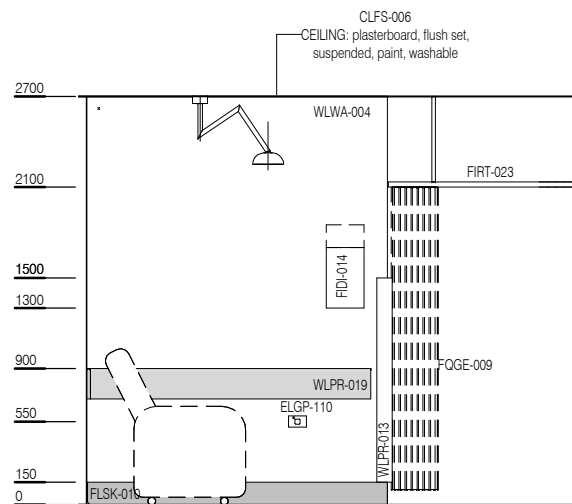
ELEVATION 2
