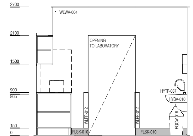
ELEVATION 2
