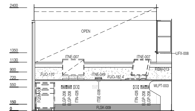
ELEVATION 4
