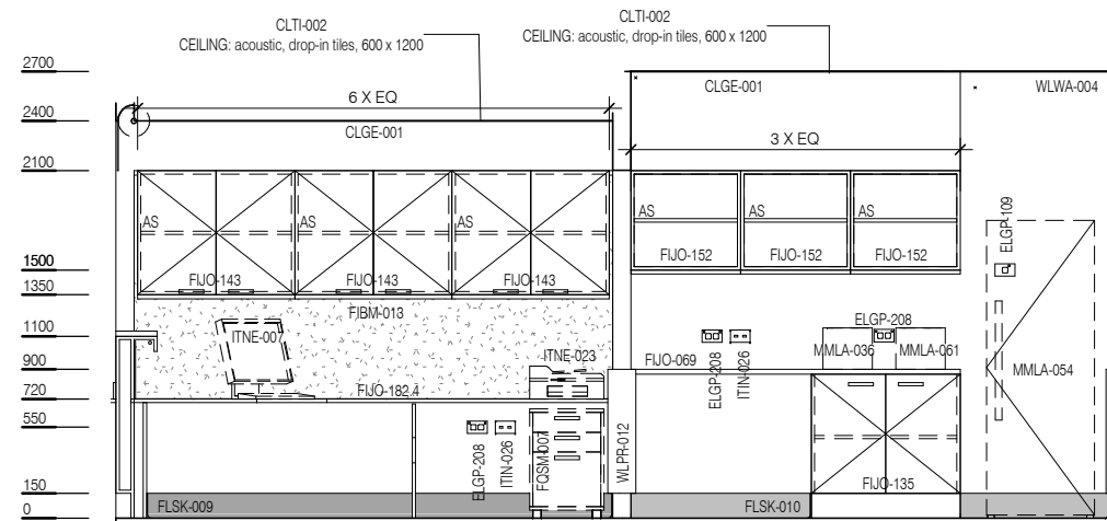
ELEVATION 1
