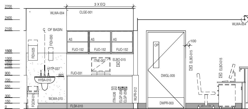
ELEVATION 3
