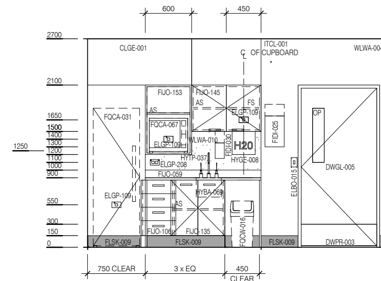
ELEVATION 3
