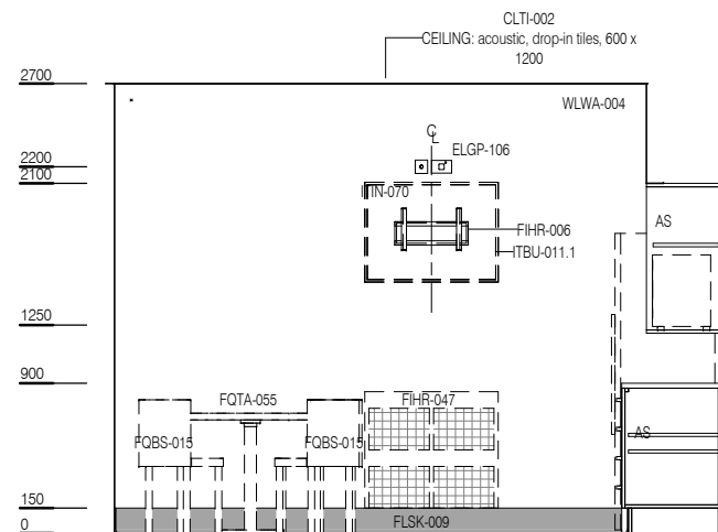
ELEVATION 2
