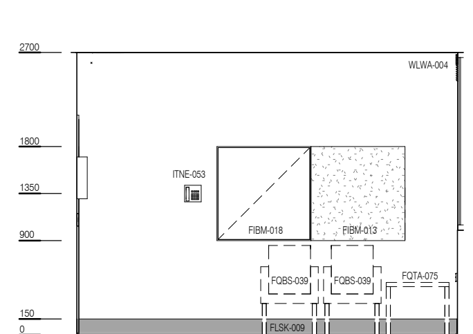
ELEVATION 4
