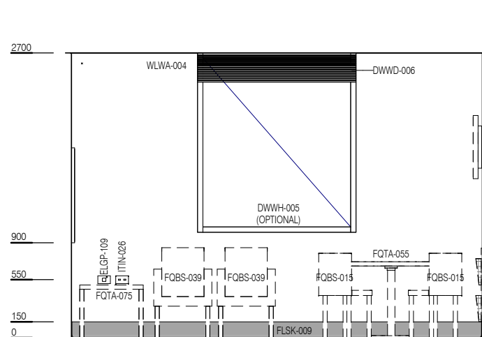
ELEVATION 1
