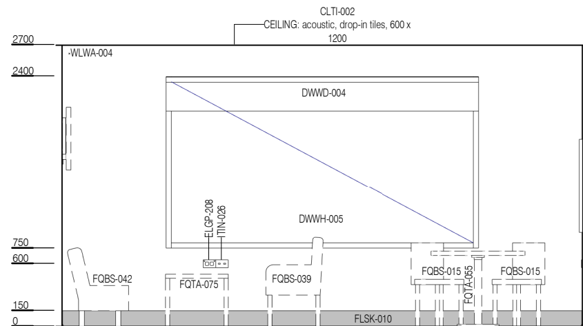
ELEVATION 1
