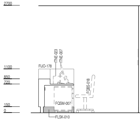
ELEVATION 1
