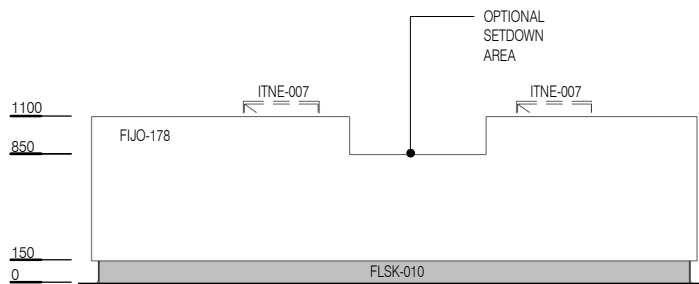
ELEVATION 5
