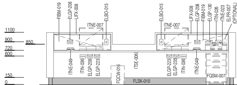
ELEVATION 4
